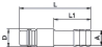
Einstecktülle
