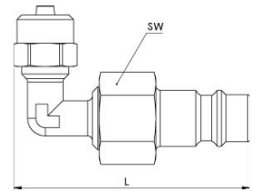
Einsteckwinkel
